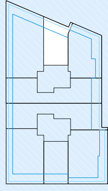
APPARTEMENT 4 PIÈCES (GE) PLAN TYPE - DUPLEX EST HAUTEUR SOUS-PLAFOND : 2,50 m
